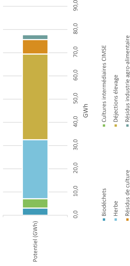
Potentiel de production d'énergie renouvelable par méthanisation en 2050 - Terre d'Emeraude (GWh)
