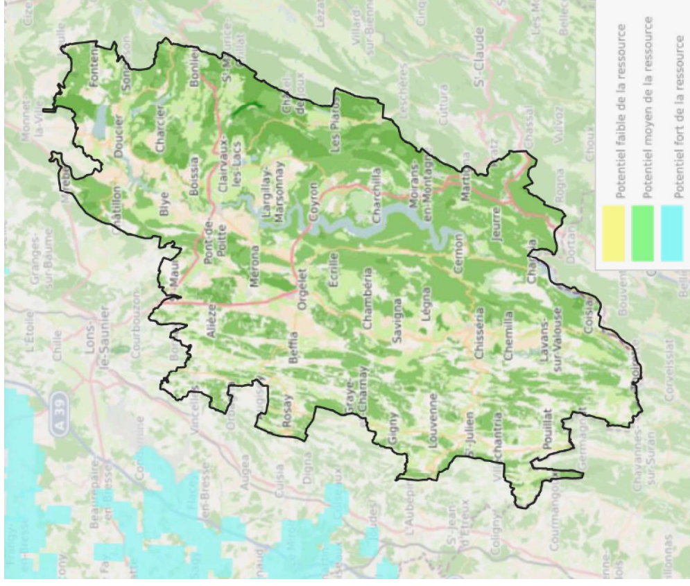
Ressources géothermales de surface en Bourgogne-Franche-Comté (source : geothermies.fr )
